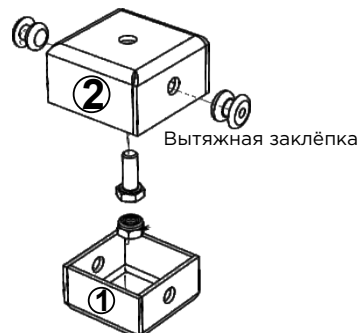
Вытяжная заклёпка
